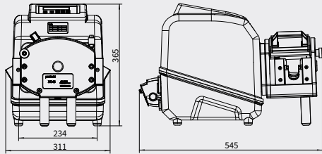
外形尺寸图
