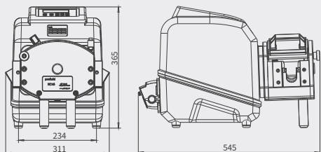
外形尺寸图
