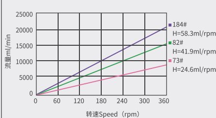
TH35流量曲线图
