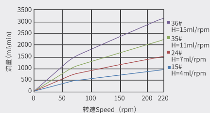
TH25流量曲线图
