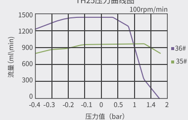
TH25压力曲线图
