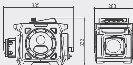
外形尺寸图
