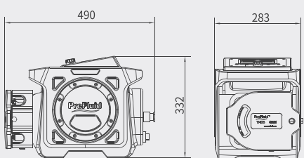
外形尺寸图
