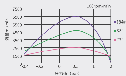
TH35压力曲线图
